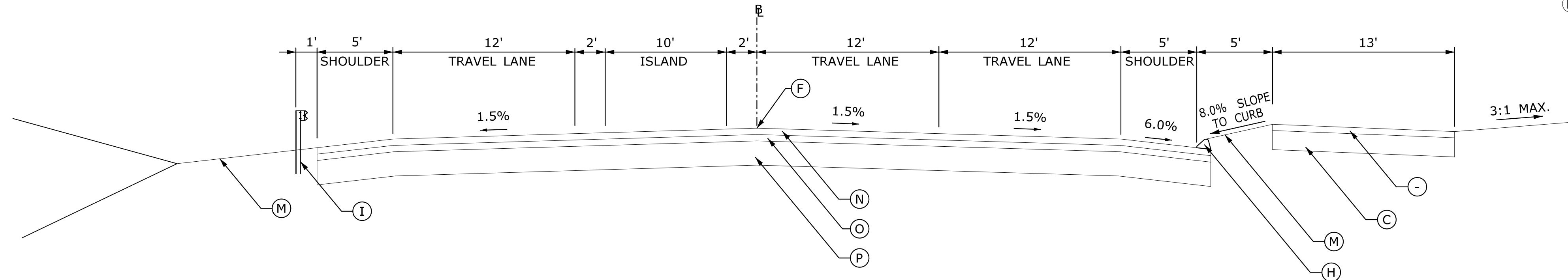
NEW BRITAIN AVENUE ROADWAY SECTION STA. 69+00 ± N.T.S.
